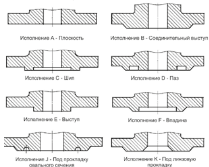
Исполнение фланца по ГОСТ 33259-2015
