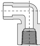
Фитинг угловой проходной под приварку внахлест с внутренней резьбой RizurLok-P-W-Pf
